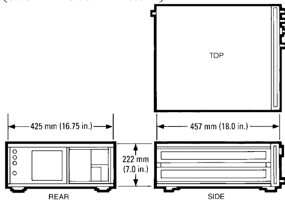
HP 8753ET/ES physical dimensions
